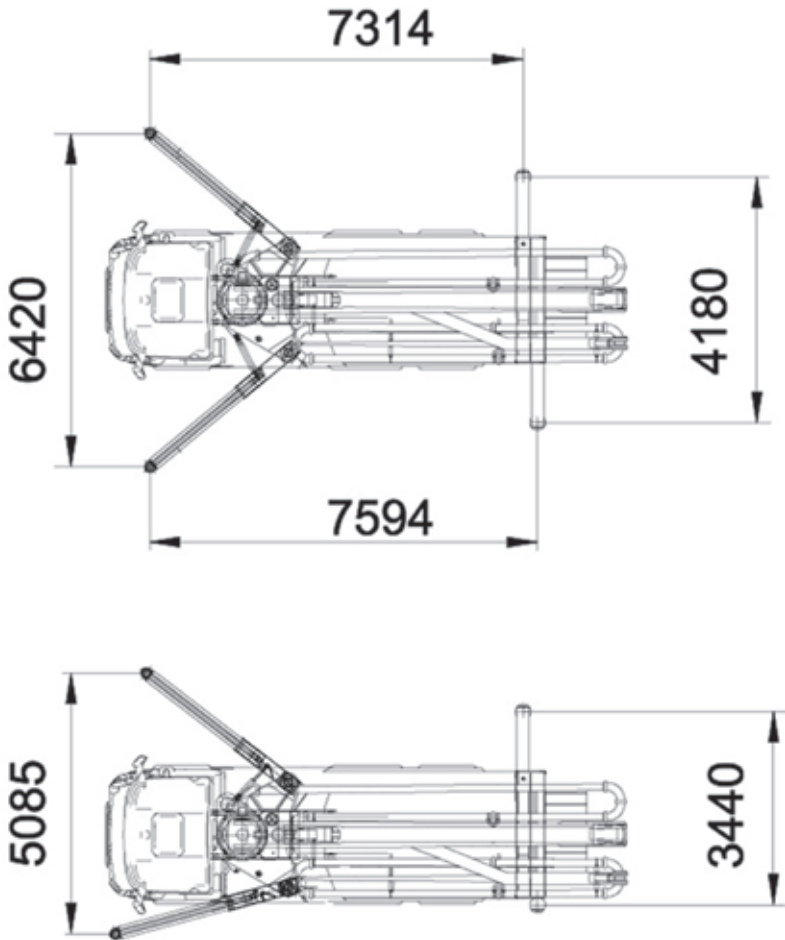
Eingeschränkter Arbeitsbereich bei einseitigem Aufbau
