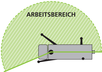
Eingeschränkter Arbeitsbereich bei einseitigem Aufbau
